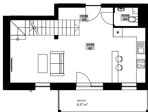
RZUT III PIĘTRA
