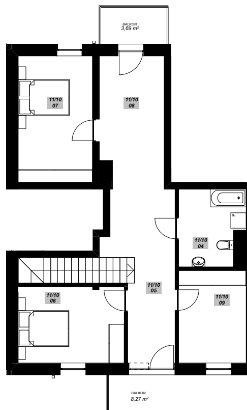
RZUT PODDASZA
