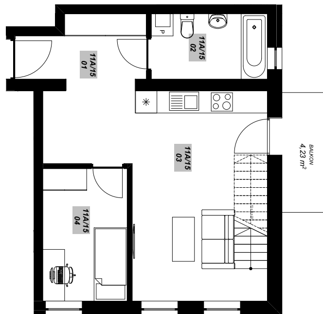
RZUT III PIĘTRA
