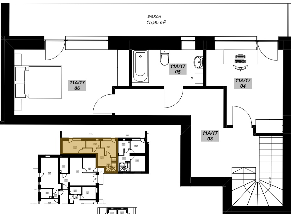
RZUT I PIĘTRA
