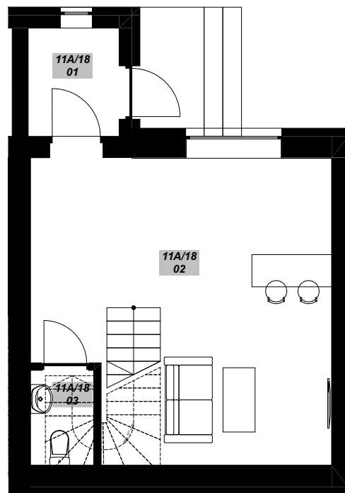
RZUT PARTERU
